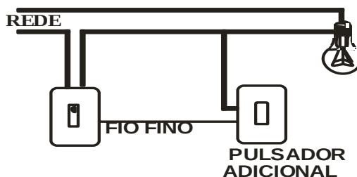
LIGAÇÃO PARALELA (2 OU MAIS PONTOS DE ACIONAMENTO ) USANDO PULSADORES ADICIONAIS
